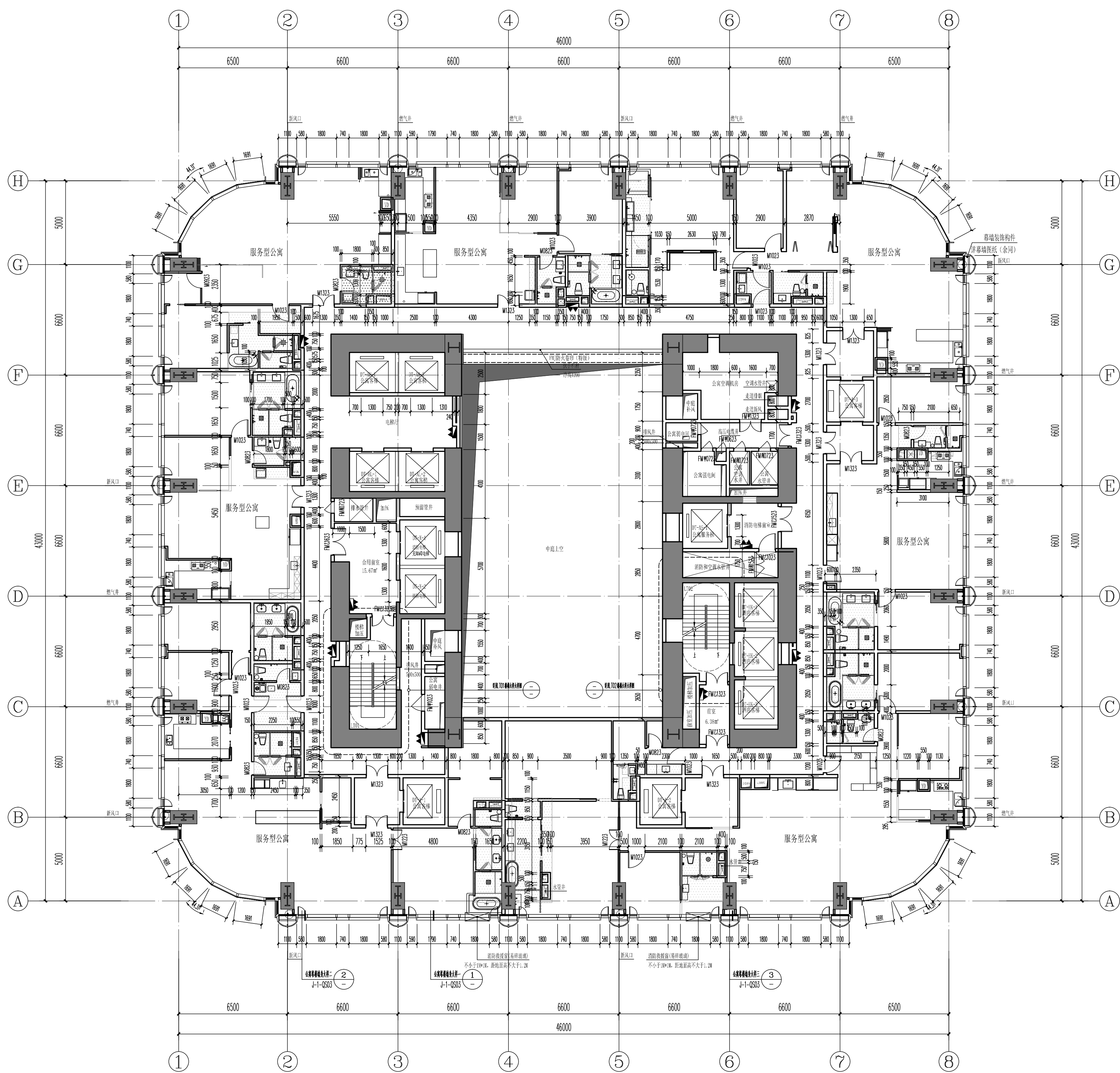
七~十三层平面图 1:150
